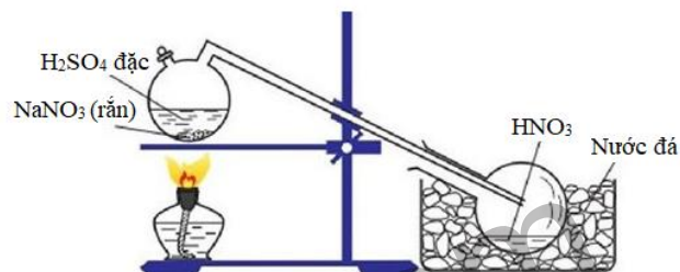
Thí nghiệm điều chế \text{HNO}_3
